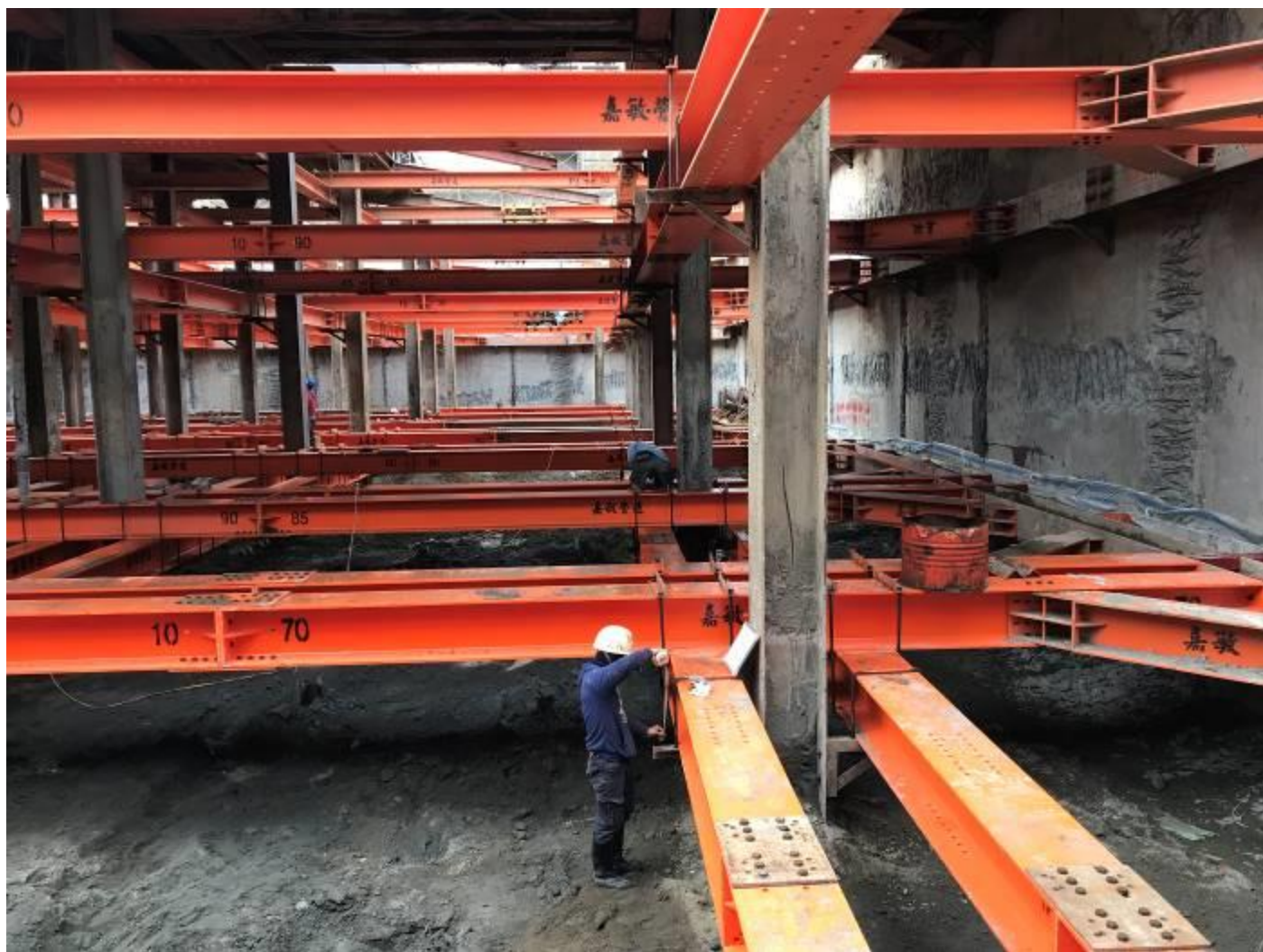
1111230 第三層水平支撐
