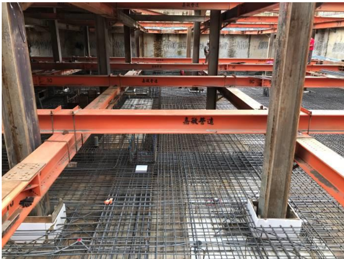
B2 鋼筋綁紮完成 1120627
