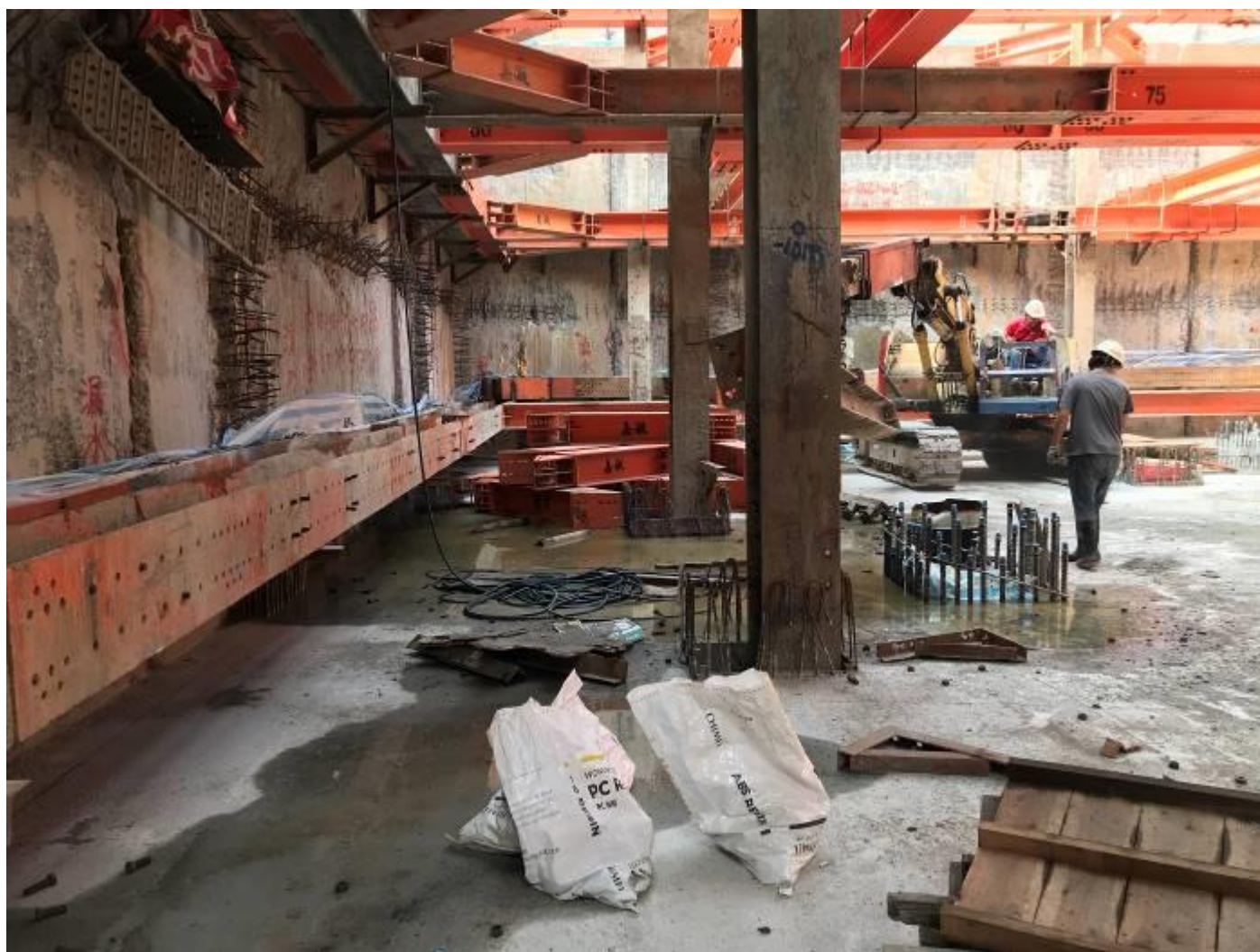
B4 安全支撐拆除 1120418
